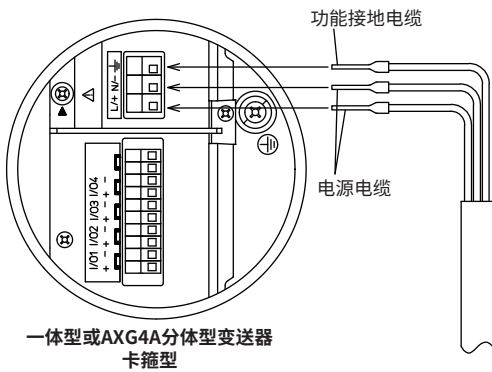
用于EtherNet/IP通信型的 一体型或AXG4A分体型变送器 M4螺丝型
