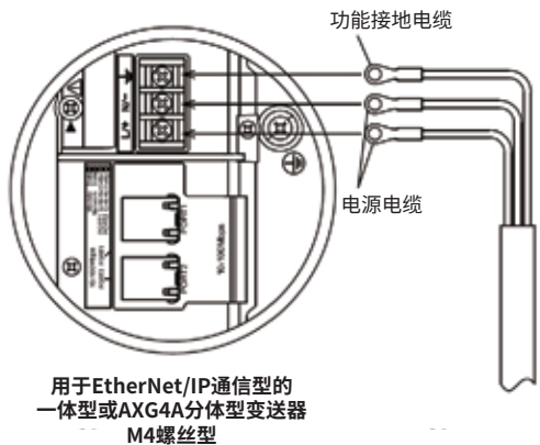
一体型或AXG4A分体型变送器 M4螺丝型
