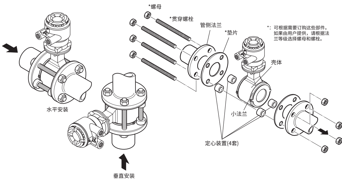
图3.3.4 夹持型的安装步骤(口径:50~200 mm (2~8 in.))
