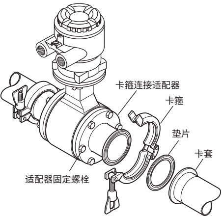
图3.3.6 卡箍型安装步骤
