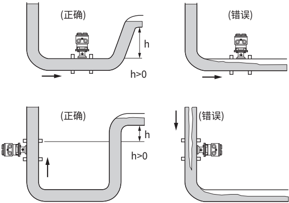
图3.1.4 安装位置
