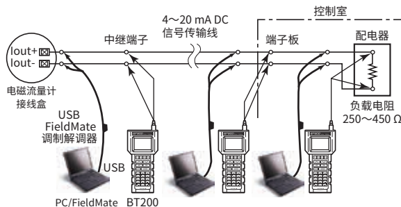
图5.6 连接BRAIN配置工具
