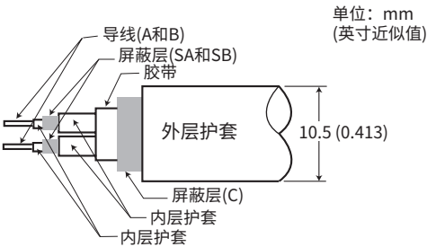
图4.2.2 专用信号电缆
