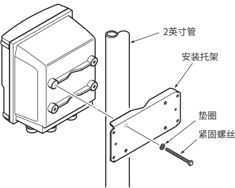
图3.4.4 2英寸管安装
