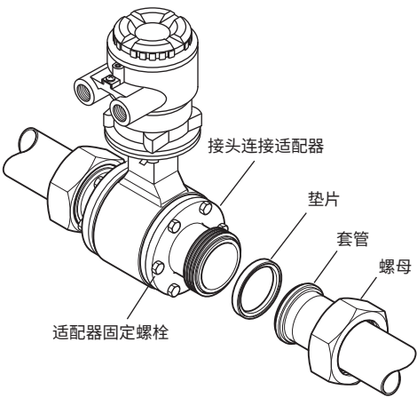
图3.3.7 接头型安装步骤
