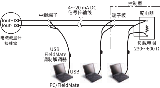
图5.7 连接HART配置工具
