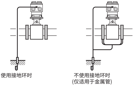
图4.5.6 接地(分体型传感器)
