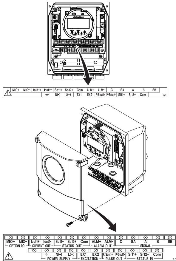
图4.4.11 端子配置(AXG1A分体型变送器)
