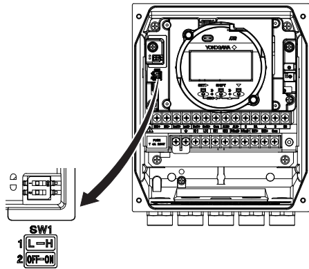
图6.3.4 硬件开关
