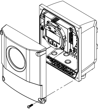
图6.3.3 移除壳盖
