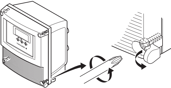
图4.4.12 取下前盖(AXFA11分体型变送器)
