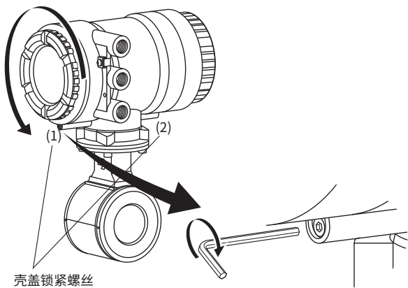
图4.4.6 取下一体型流量计的接线盒盖
