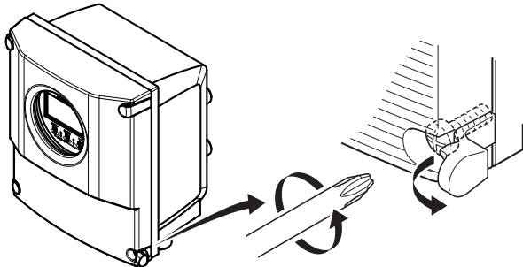
图4.4.10 取下前盖(AXG1A分体型变送器)
