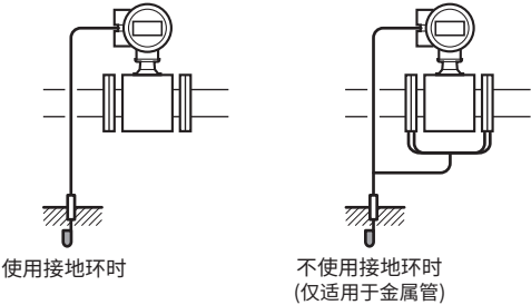
图4.4.5 接地(一体型流量计)
