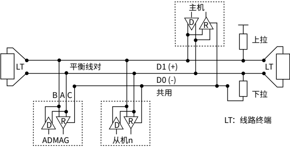
图6.3.2 Modbus连接
