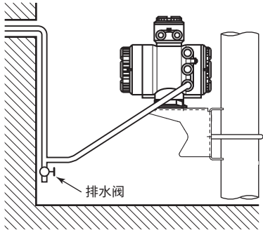
图4.3.3 分体型变送器(AXG4A)
