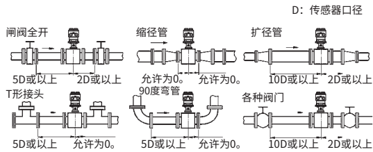
图3.1.1 直管段所需长度
