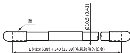
图4.2.3 信号电缆的电缆终端
