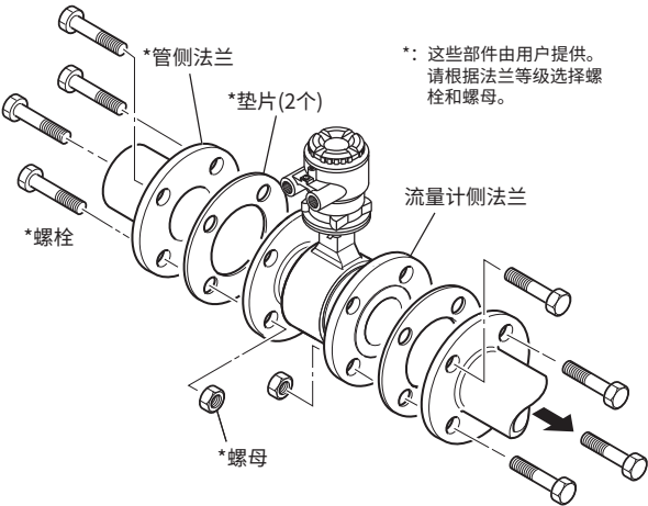
图3.3.5 法兰型的安装步骤(口径:2.5 ~ 500 mm (0.1 ~ 20 in.))
