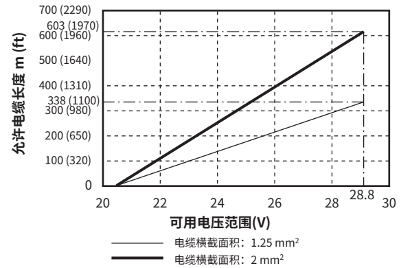
图4.4.2 供电电压和电源电缆长度(一体型流量计和AXG4A分体型变送器)
