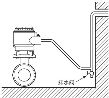
图4.3.2 分体型传感器
