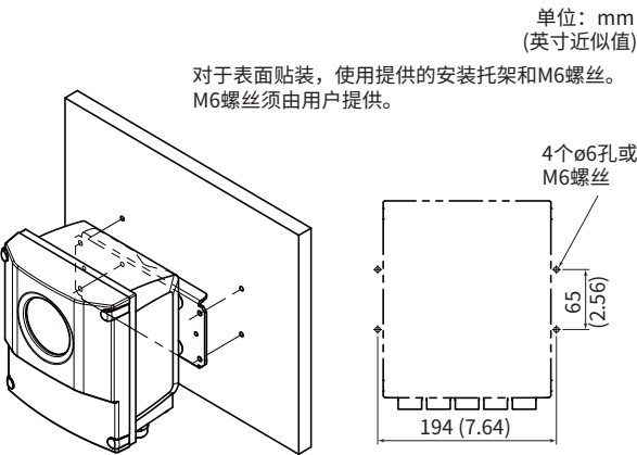
图3.4.3 表面贴装
