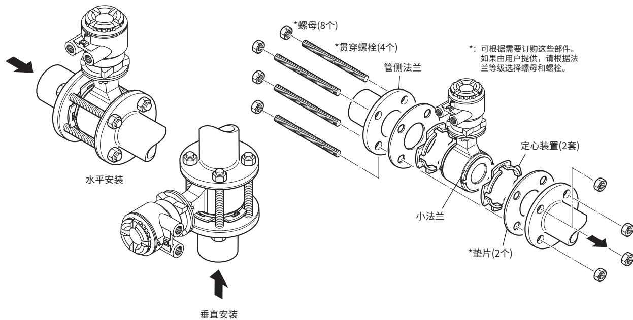
图3.3.3 夹持型的安装步骤(口径:25~40 mm (1~1.5 in.))
