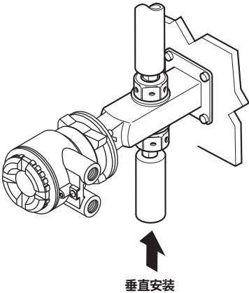
图3.3.1 组合接头型的安装步骤 (口径:2.5 ~ 10 mm (0.1 ~ 0.4 in.))
