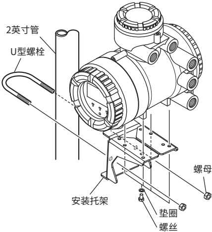
图3.4.1 2英寸管垂直安装
