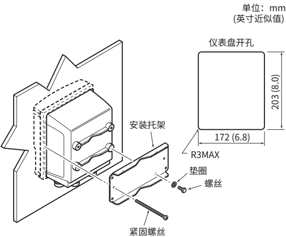
图3.4.5 盘装
