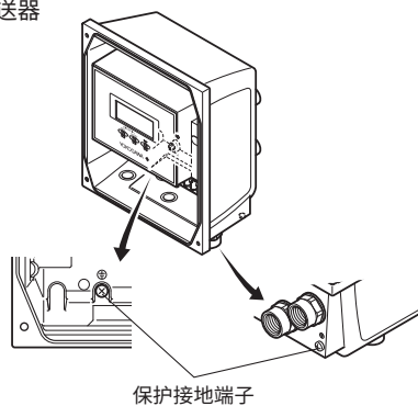
图4.4.4 保护接地端子的位置
