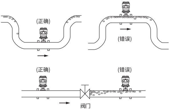
图3.1.5 避免气泡
