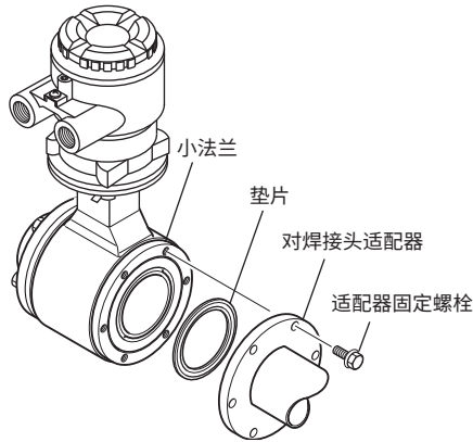
图3.3.8 对焊接头型安装步骤
