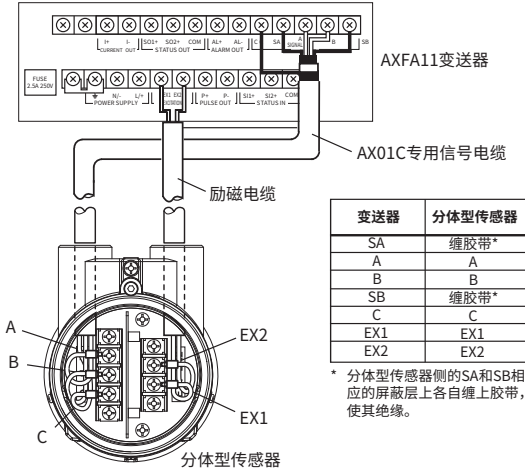
图4.5.5 接线图(AXFA11分体型变送器)
