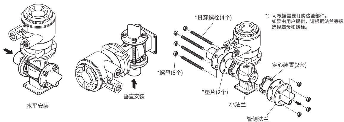
图3.3.2 夹持型的安装步骤(口径:2.5~15 mm (0.1~0.5 in.))
