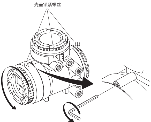
图4.4.7 取下AXG4A分体型变送器的接线盒盖
