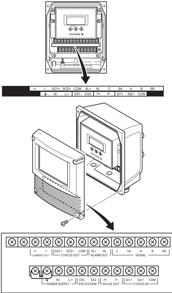
图4.4.13 端子配置(AXFA11分体型变送器)
