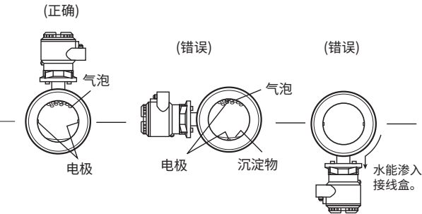
图3.1.6 安装方向
